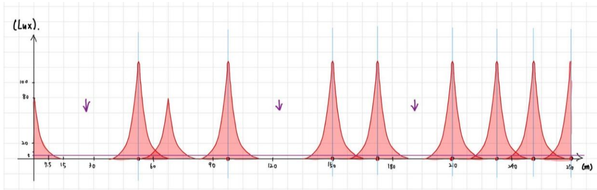
(圖 6-3) 路燈亮度與路徑剖面圖(研究者自行繪製)。
