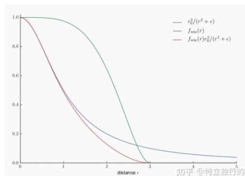
(圖 3) 聚光燈之照明模型示意圖(研究者自行繪製) (圖 4) 三種距離衰減函數模型示意圖(研究者自行繪製)。
