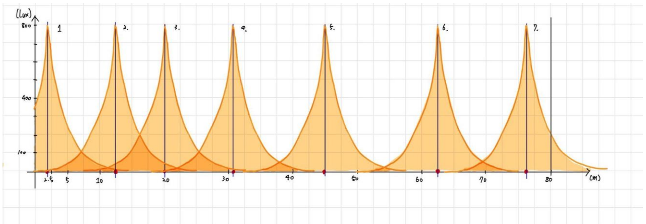
(圖 9-5) 改善後路燈亮度與路徑剖面圖(研究者自行繪製)。
