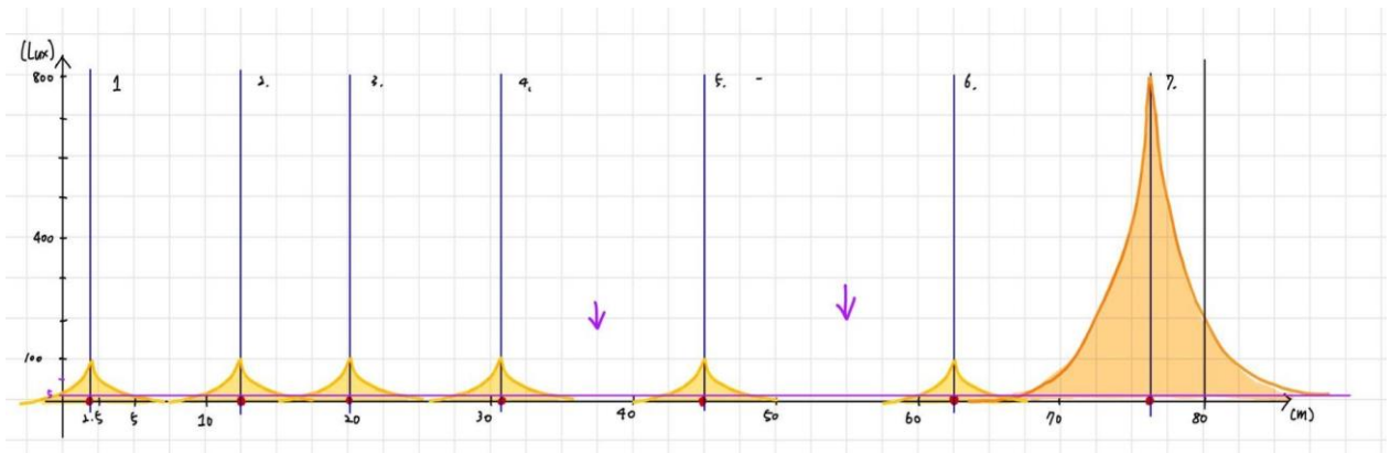
(圖 9-4) 改善前路燈亮度與路徑剖面圖(研究者自行繪製)。
