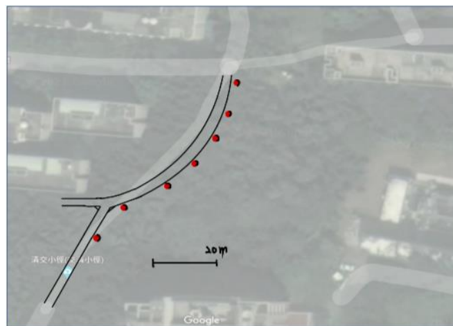
(圖 9-1) 路燈地理位置分布圖(研究者自行繪製)。
